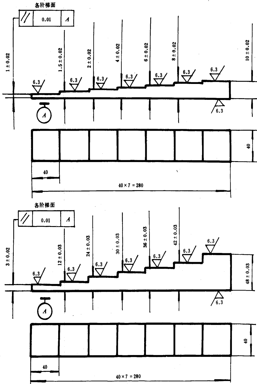
图 2 试块
